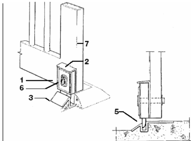
Vertikální upevnění (dvě křídla)
